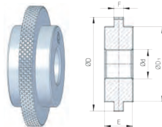
Moleta escalonada (dos caras) Stepped knurl (two sides)
