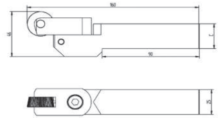
Modelo M15 25
